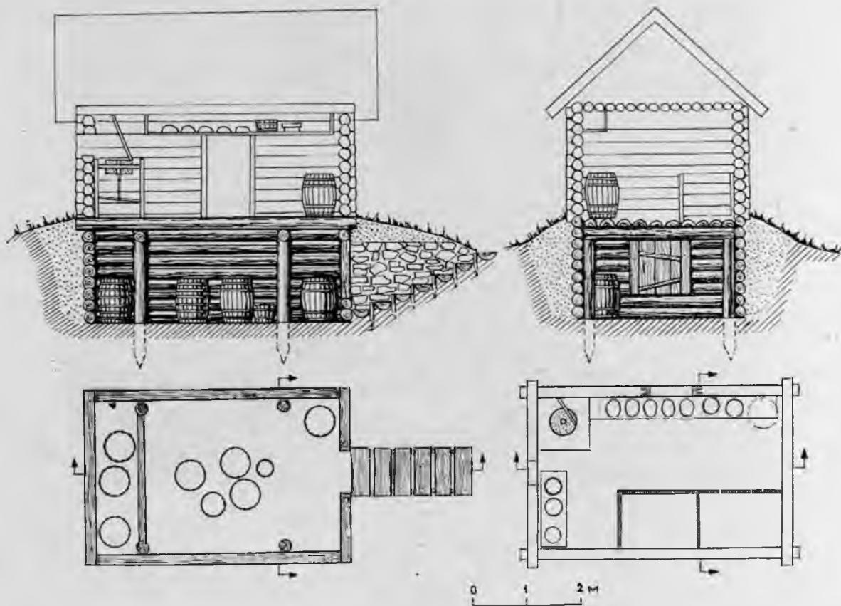
141. att. 19. laukuma saimniecības celtne (rekonstrukcija).
