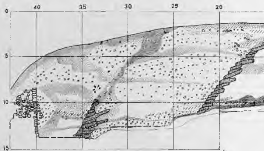
102. att. Sēlpils priekšpils. 1 — F laukuma rietumu profils, 2 — grāvja (G laukuma) rietumu profils.
