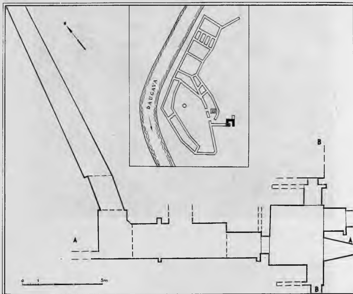
49. att. Torņa uzmērojuma shēma. Ietvarā — Sēlpils pilskalna plāns ar melni iezīmētu torni Pauluči albumā.
