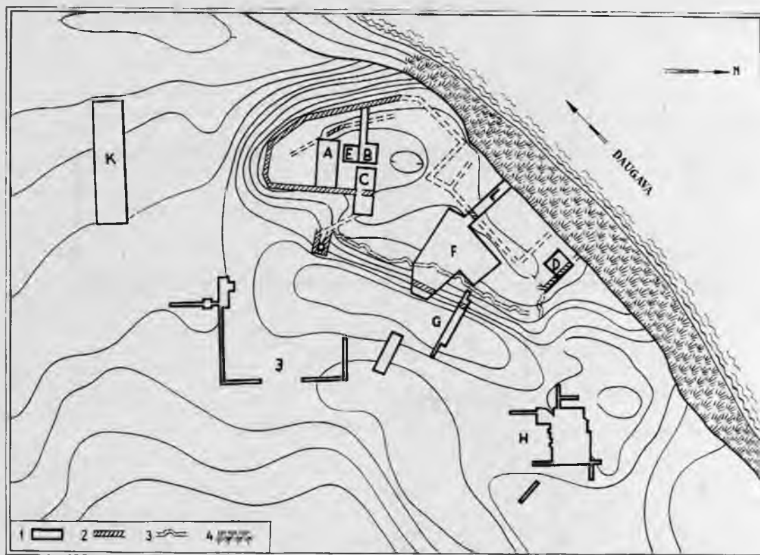
7. att. Sēlpils pilskalna un izrakumu plāns: A, B, C, E — plankums, D, L, F, G — priekšpils, K, J — apmetne, H — kapsēta. 1 — izrakumu laukumi, 2 — mūris, 3 — kara laika tranšejas, 4 — krasta krauja
