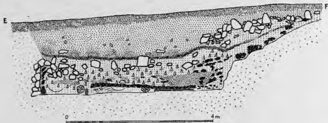
132. att. Jā laukums, celtnes vietas griezumšs.
